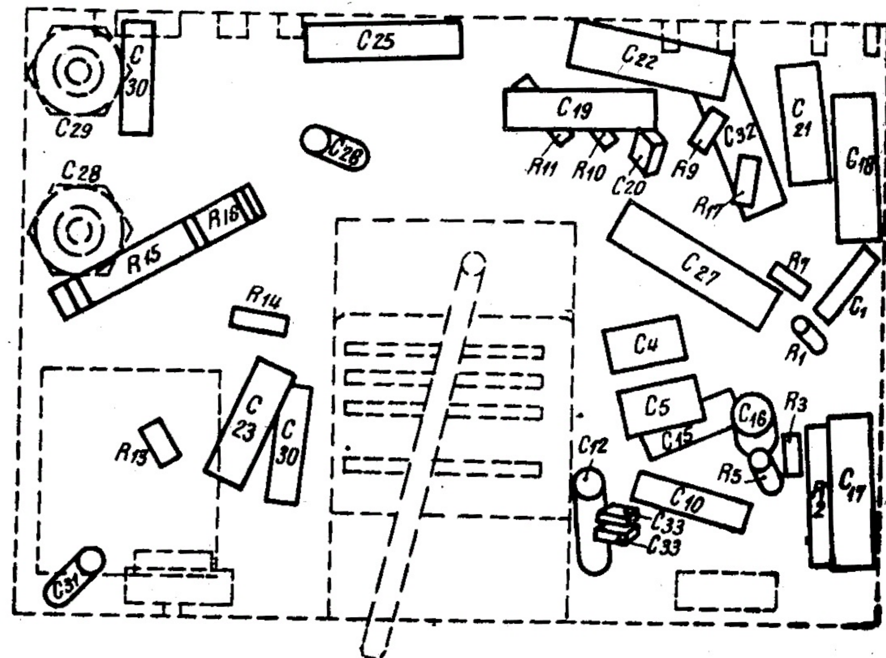
Disposition des éléments à l'intérieur du châssis.
